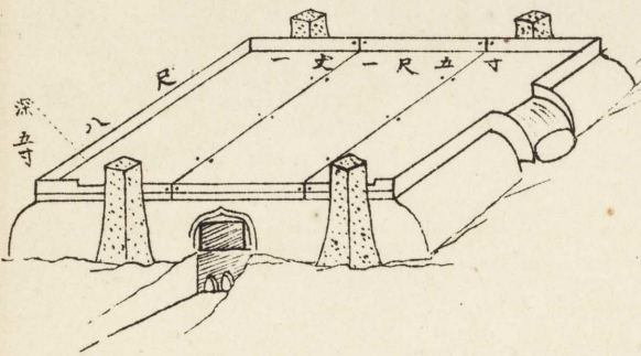
鐵釜之圖
