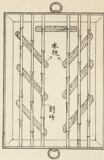
沼井之構造
