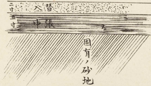
地盤断面圖
