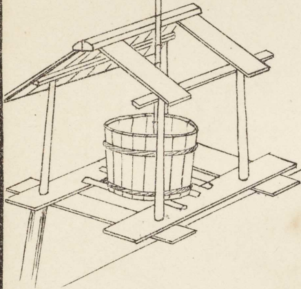
海水汲揚装置圖
