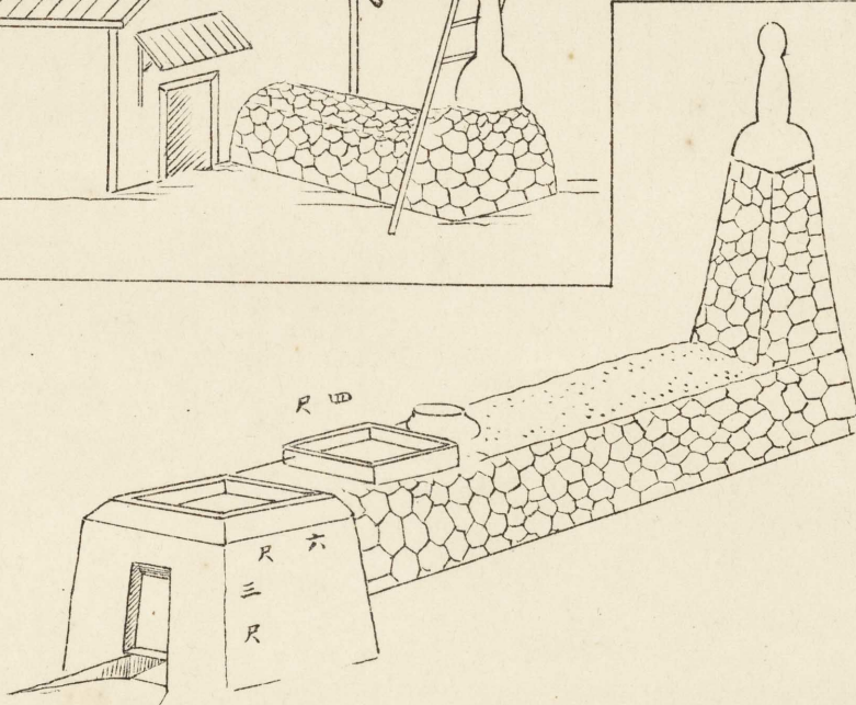
釜屋(二)
