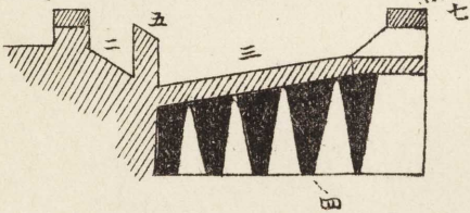
全(断面)
