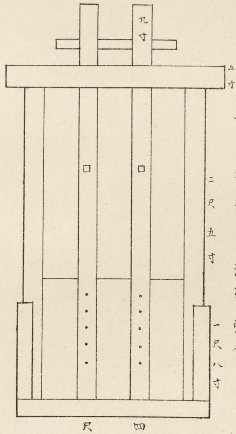
水間正面
