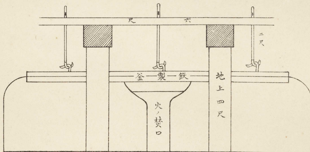
圖面正、釜。竈
