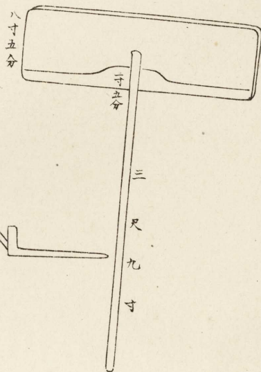
よせ鍬
