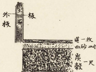
散鹽貯藏場地下構造
