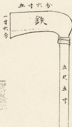
ふちきり鎌
