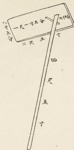
へりいれ
