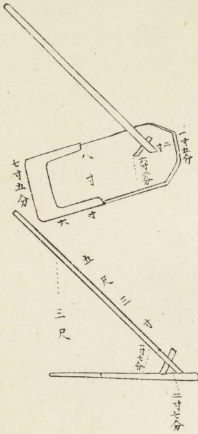
沼井堀鋏
