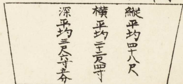
鹹水貯藏池
