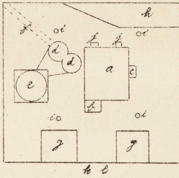
入口 釜柱 燃料置場 煙出し 出湯場 温ノ釜 釜焚口 竈
