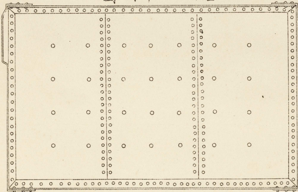
鐵釜(鍛鐵)平面圖
