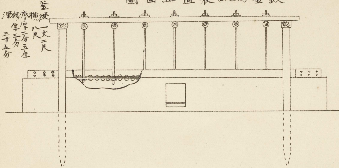
鐵釜(鍛鐵)裝置正面圖
