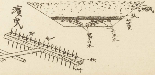
沼井装置横截圖
