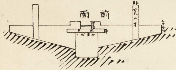
中央に於ける 横断面
