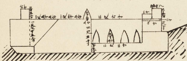
面断縦央中
