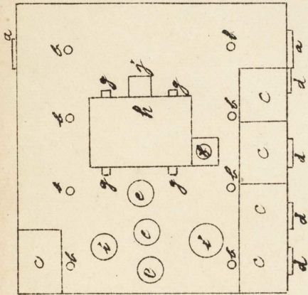
釜屋平面圖
