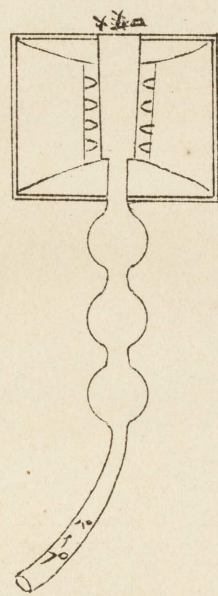
釜平面圖
