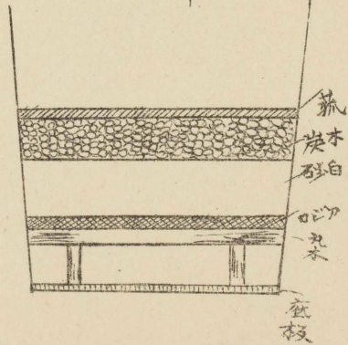
面斷縦全
