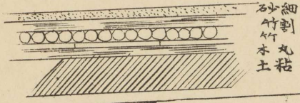
沼井前桶
