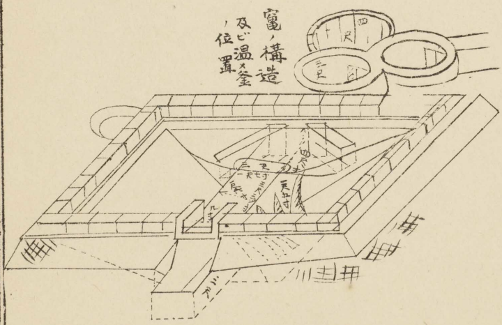
(a) 敷板 (b) 釜石 (c) 練丸 (d) 灰出口 (e) 釜口 (f) 釜肩 (g) 釣り釜
