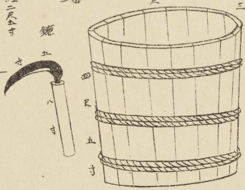
沼井穴用桶
