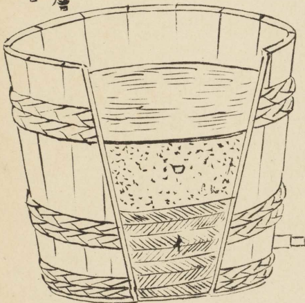
置装過沪 (上全)
