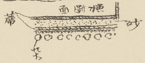
苦汁分離装置
