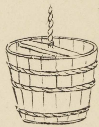
釣鉄配列方
