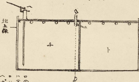
面斷 AB
