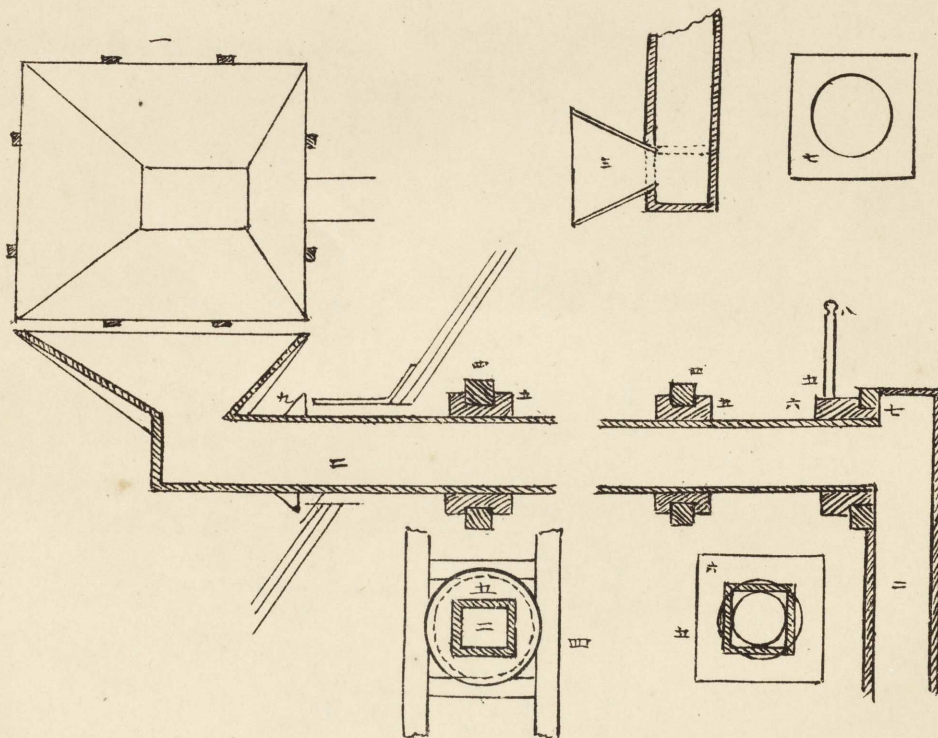
蒸發力促進裝置風取
