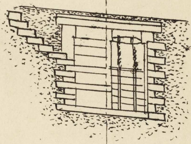
水閉正面圖
