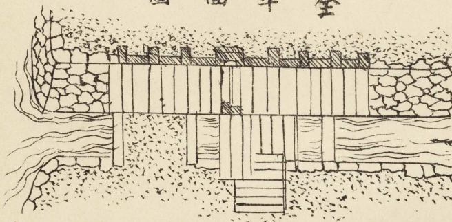
全平面圖
