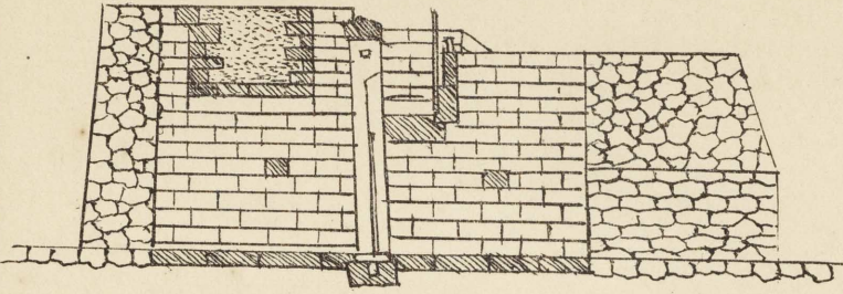
水閉側面圖
