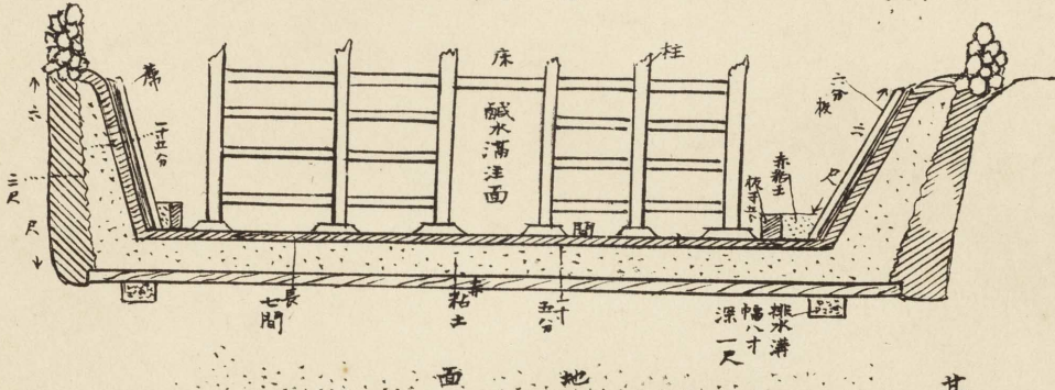
壺臺平面
