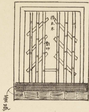
沼井構造
