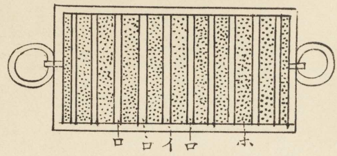
改良沼井台構造第二圖
