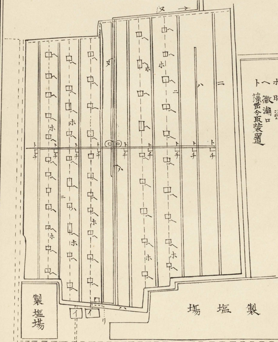
長沼井式塩田平面
