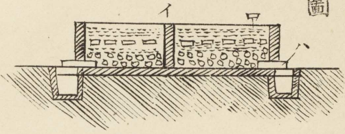
改良沼井台構造第二圖
