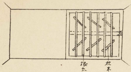
沼井内面
