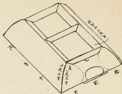
沼井外面
