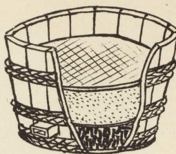
鹹水漚過装置
