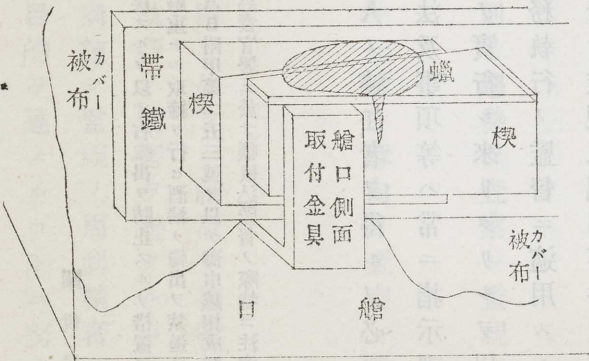
楔部断面圖及蠟封
